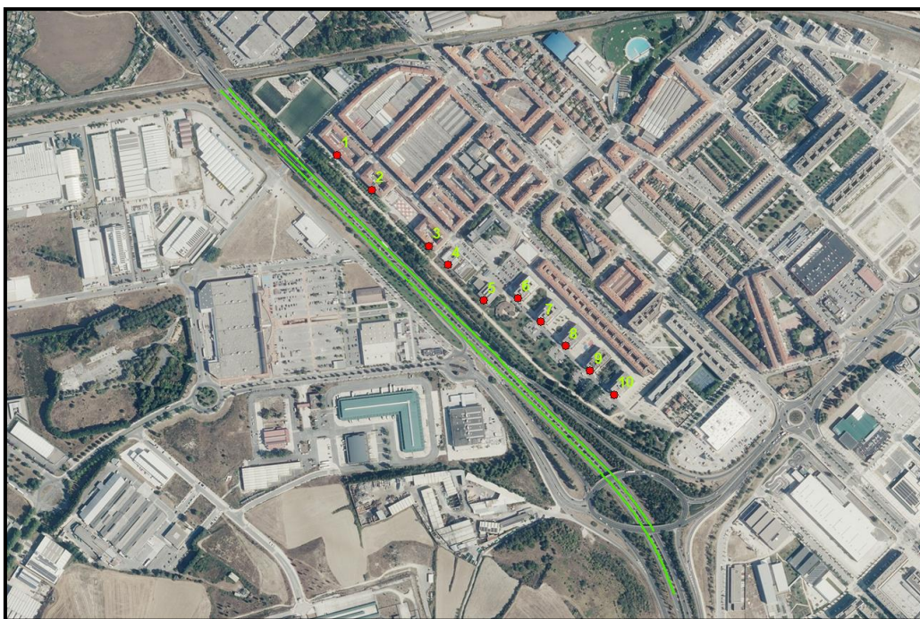
Ilustración 59. Tramos de carretera con propuesta de asfalto fonoabsorbente en el Plan Zonal 10 – Berriozar
